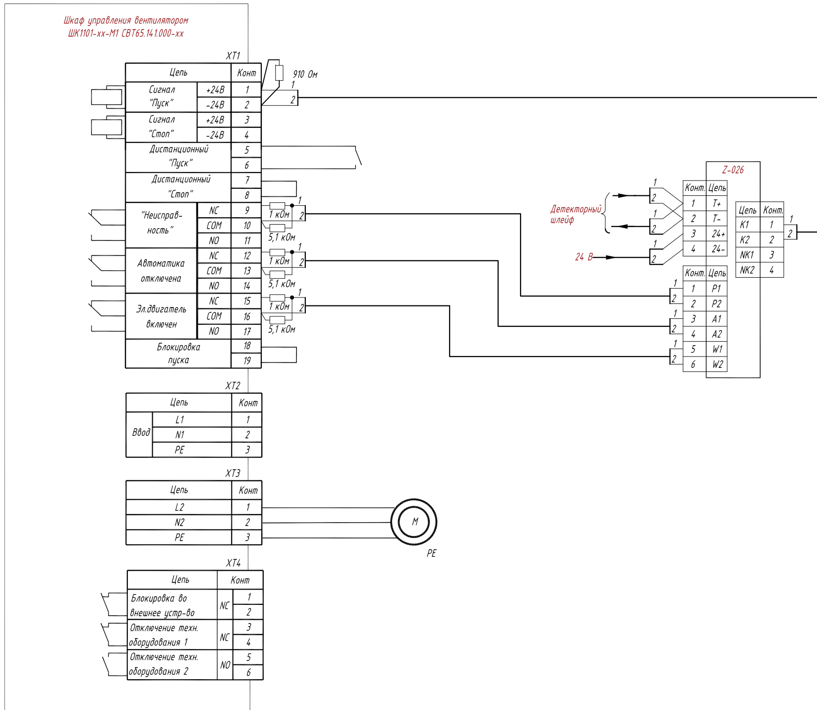
Схема подключения шкафа управления насосами ШК1101-ХХ-М1.
